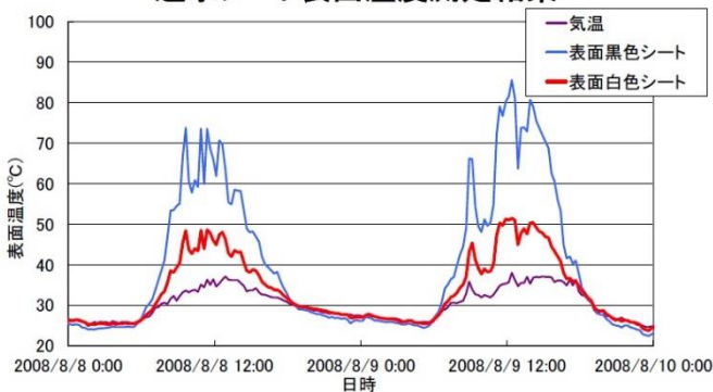
遮水シート表面温度測定結果
